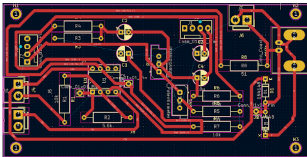
Fig. 7. Ruteo de pistas y distribución de componentes de la placa de amplificación.
